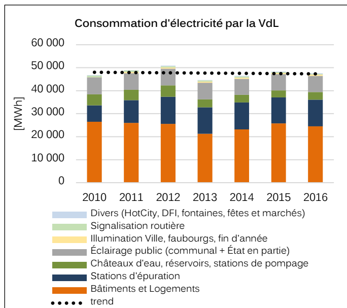
Graphique 2: Consommation d'électricité par la VdL, source: Service énergétique
