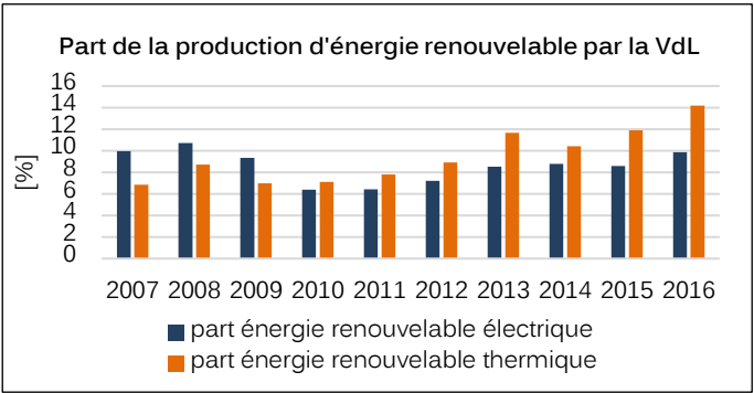
Graphique 6:Part de la production d'énergie renouvelable par la VdL à la consommation en énergie par la VdL, source: Service énergétique
