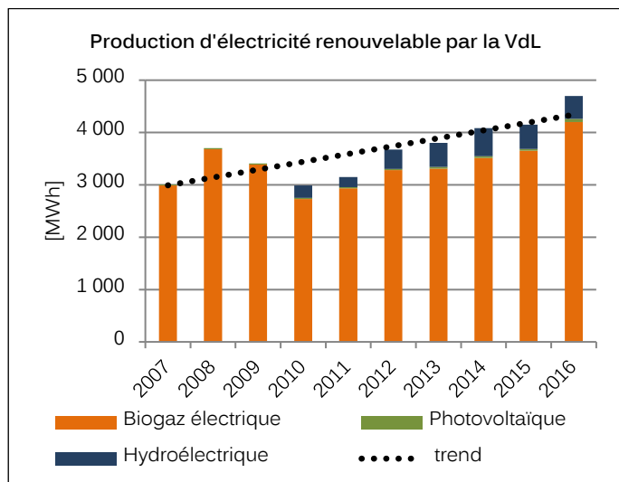
Graphique 4: Production d'électricité renouvelable par la VdL, source: Service énergétique
