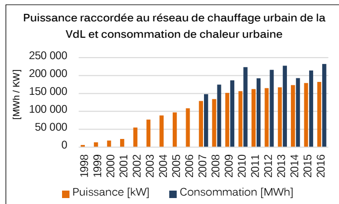
Graphique 9: Puissance raccordée au réseau de chauffage urbain de la VdL et consommation de chaleur urbaine, source : Service énergétique
