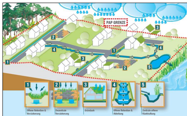
Figure 2: Exemples de rétenion et d'écoulement superficiels des eaux pluviales au sein d'un PAP, source : Leitfaden für den natürlichen Umgang mit Regenwasser in Siedlungsgebieten Luxemburgs (AGE)
