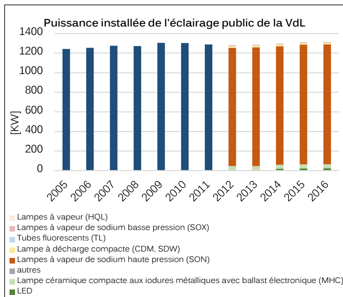
Graphique 29: Puissance installée de l'éclairage public de la VdL, source des données: Service éclairage public
