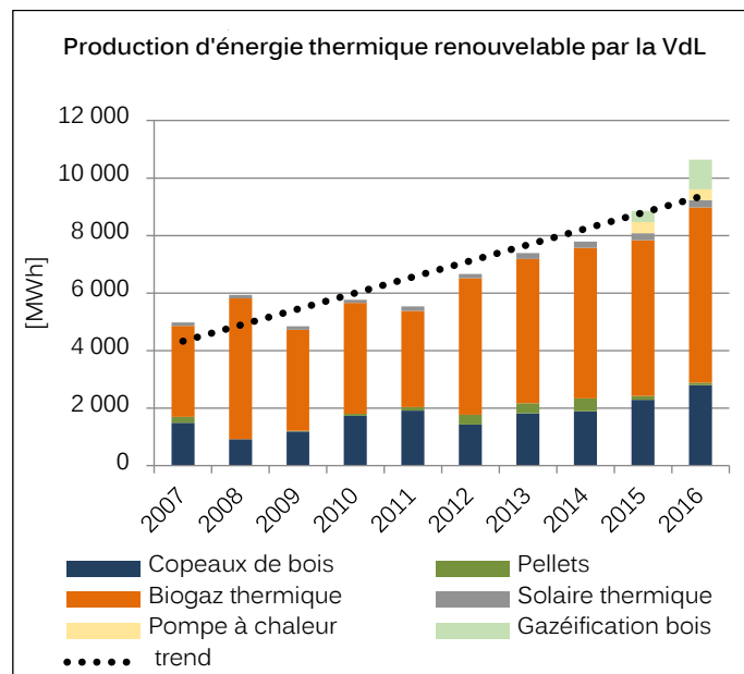
Graphique 5: Production d'énergie thermique renouvelable par la VdL, source: Service énergétique
